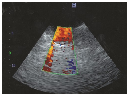
Fig. 3. Mitral regurgitation
